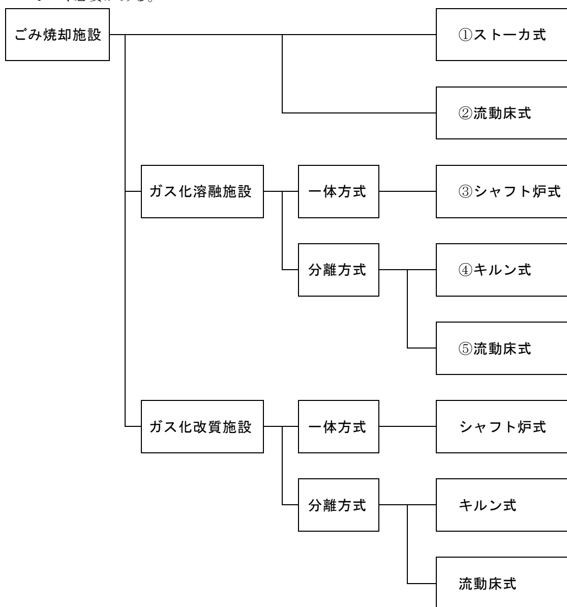
図 2.3.1 ごみ焼却施設の種類の分類
